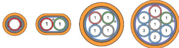
戶外直埋型 (DB-10)
