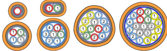
戶外直埋型 (DB-10)
